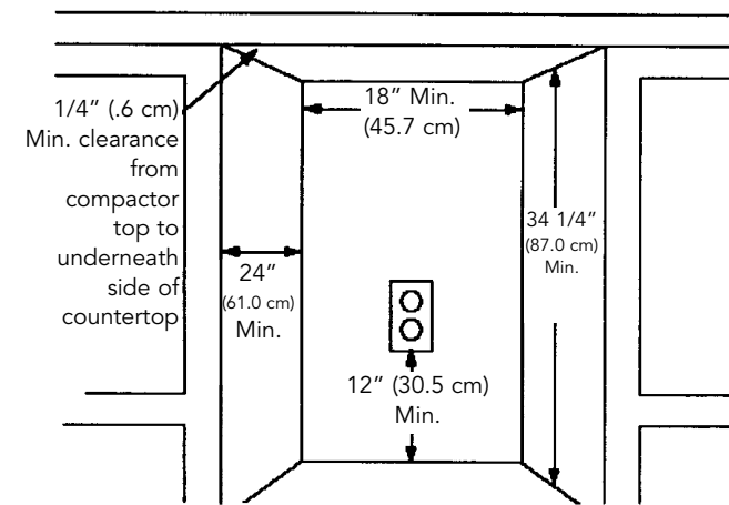
CUTOUT
